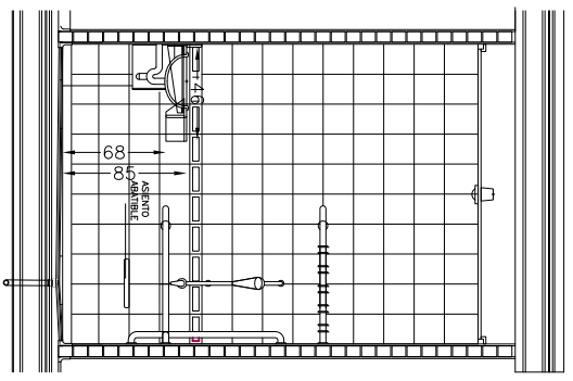
DETALLE ASEO CON DUCHA
