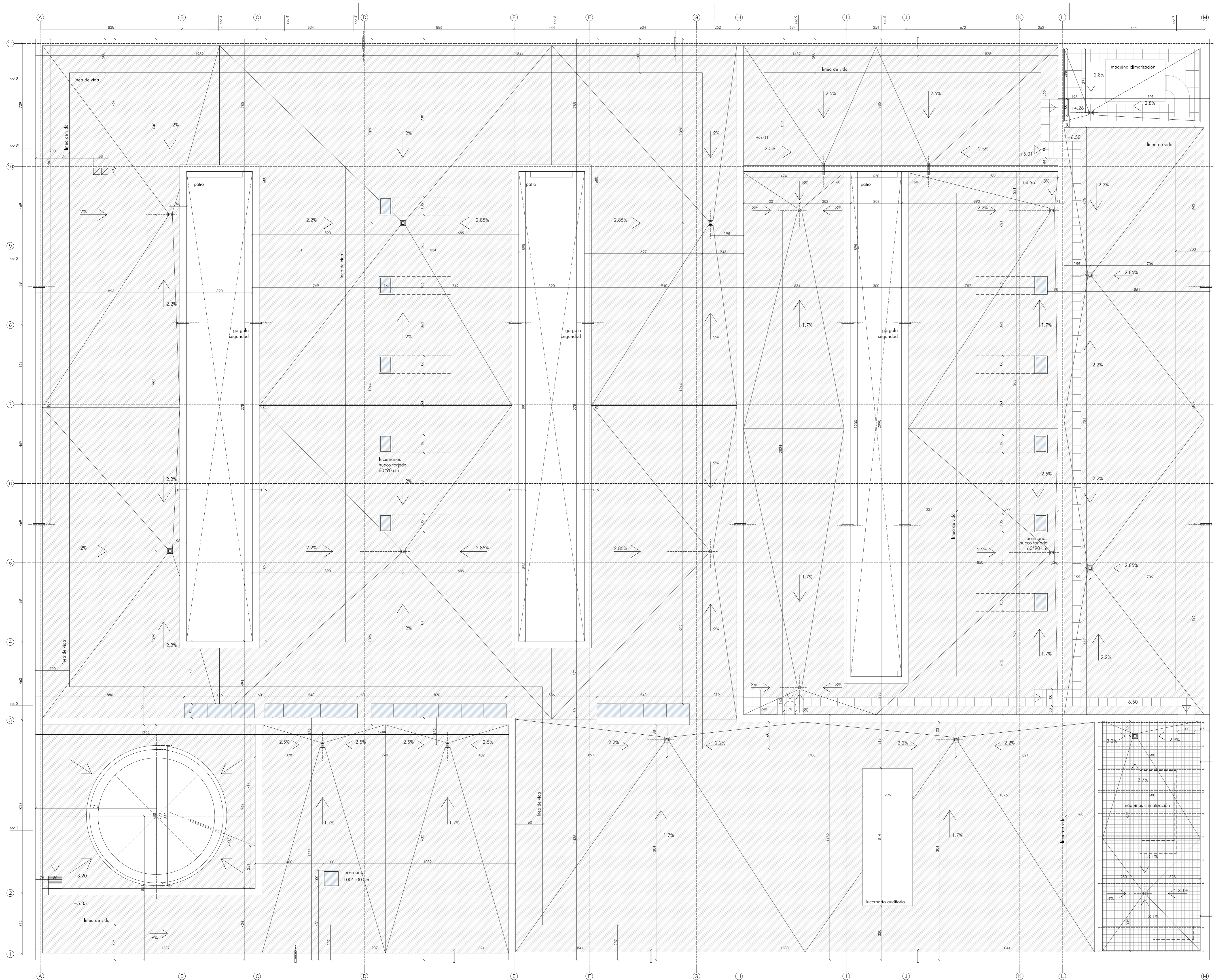
PLANTA CUBIERTA
