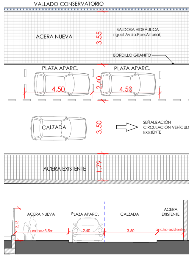
DETALLE PLANTA CALLE SECCIÓN CALLE
