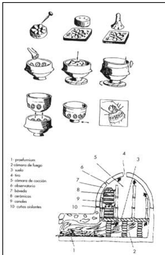
Horno cerámico romano y forma de realizar una Terra sigillata
