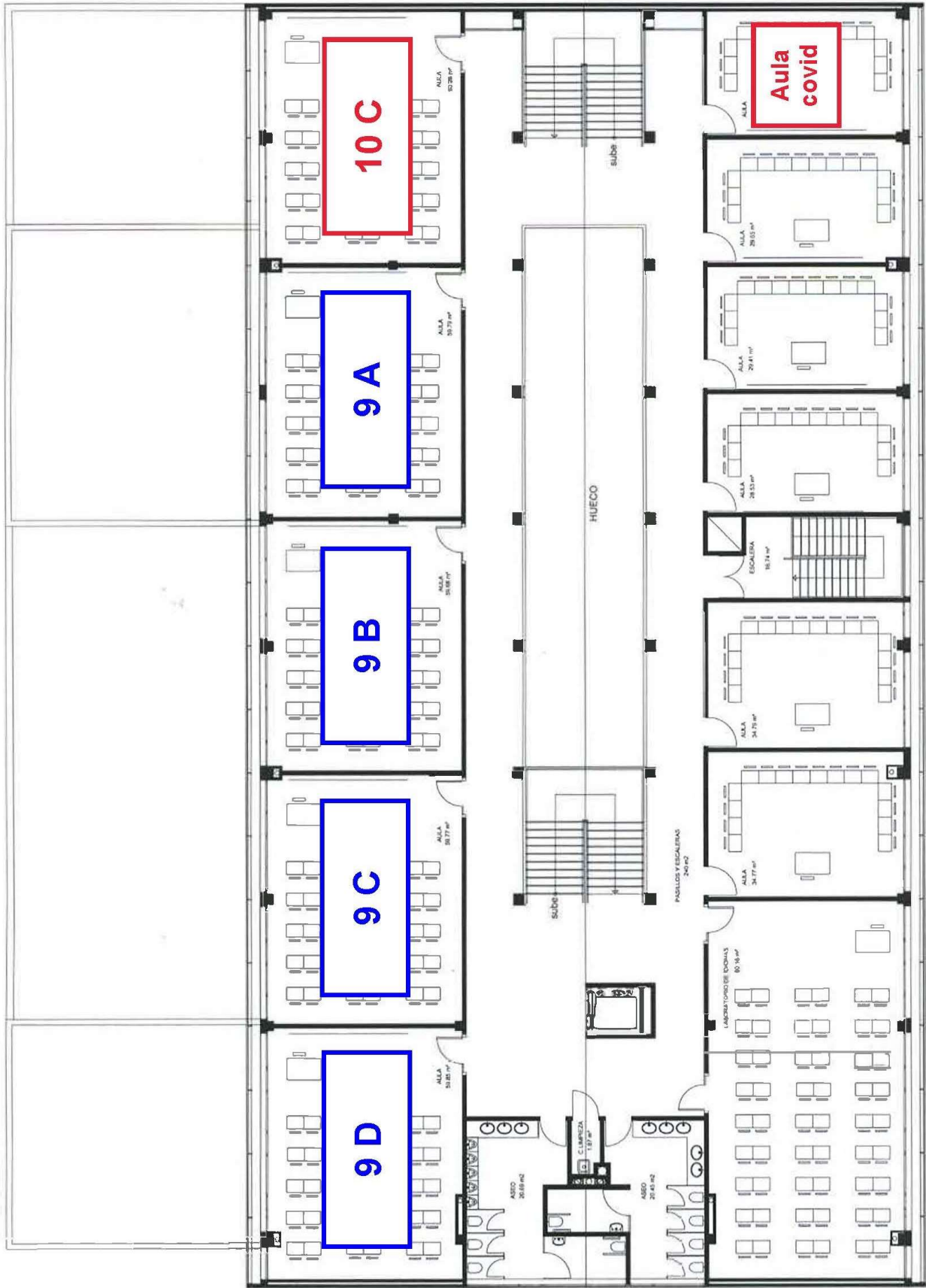
PLANTA PRIMERA SUPERFICIE CONSTRUIDA PLANTA 1 948.50 M2
