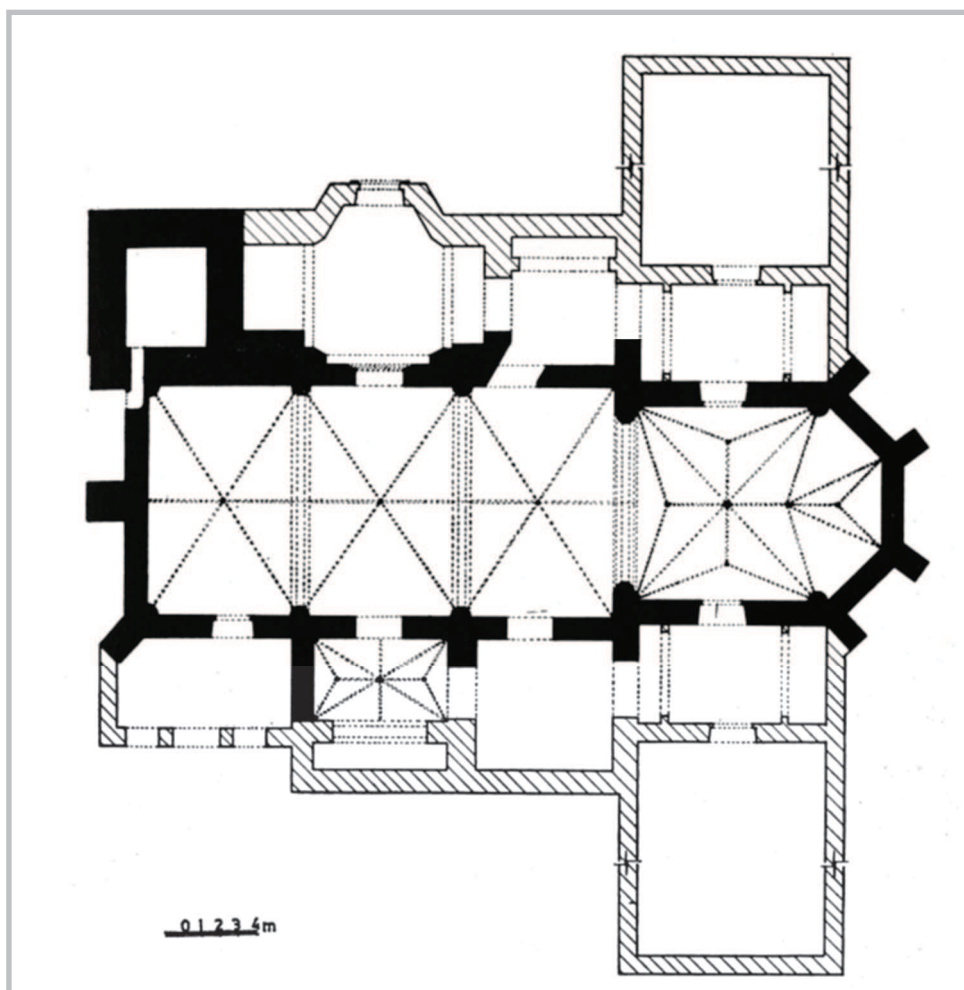
Planta de la Colegiata de Medinaceli
