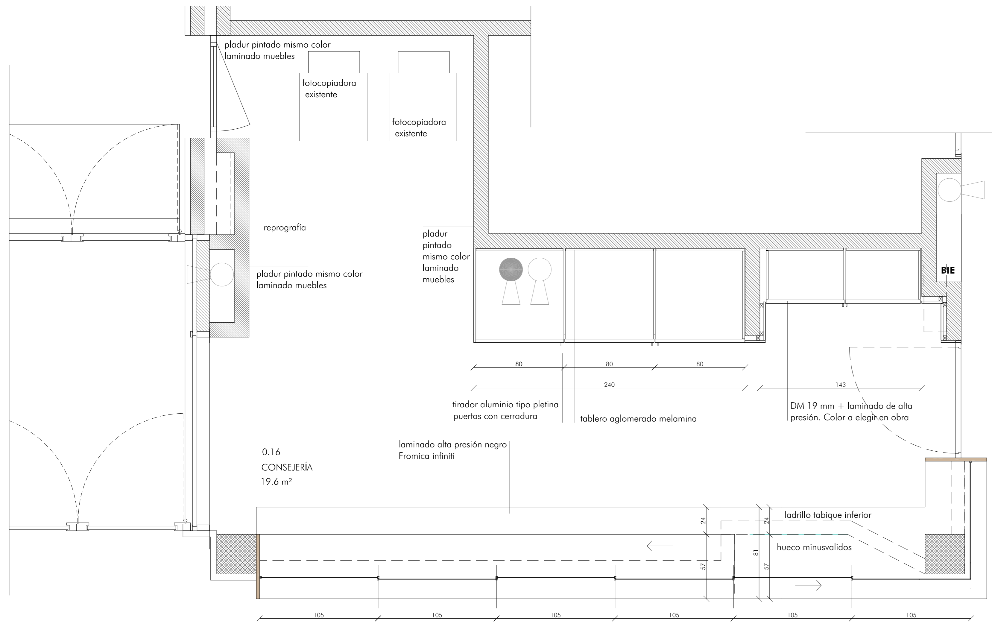
Planta conserjería. Escala 1/20
