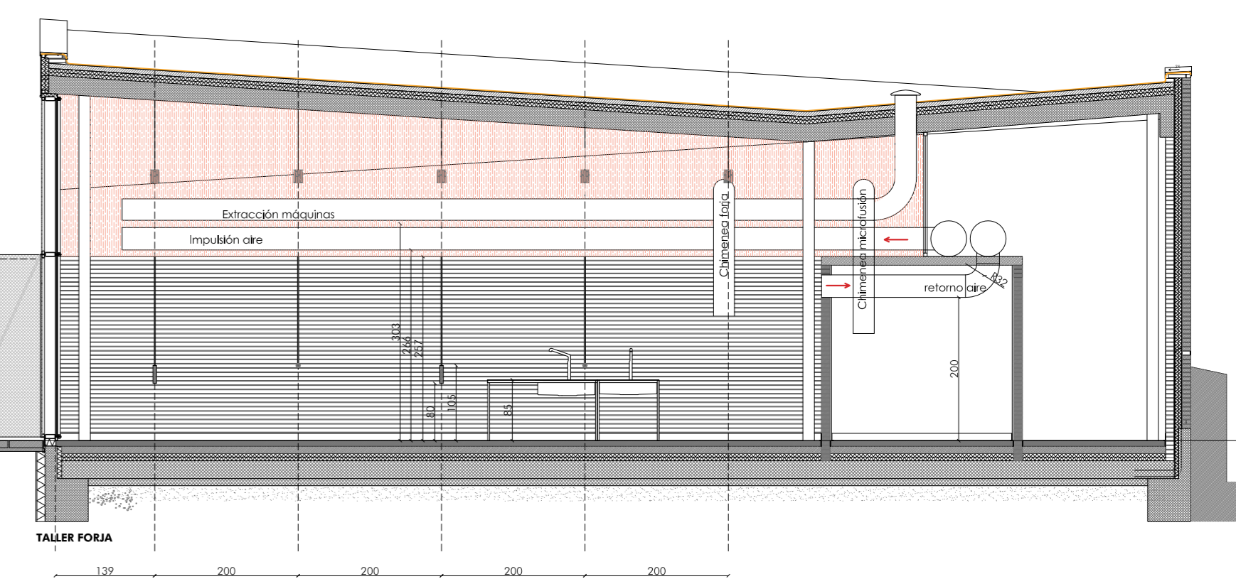
SECCIONES DISPOSICIÓN INSTALACIONES Y CONDUCTOS EXTRACCIÓN AIRE EN TALLERES. ESCALA 1:75
