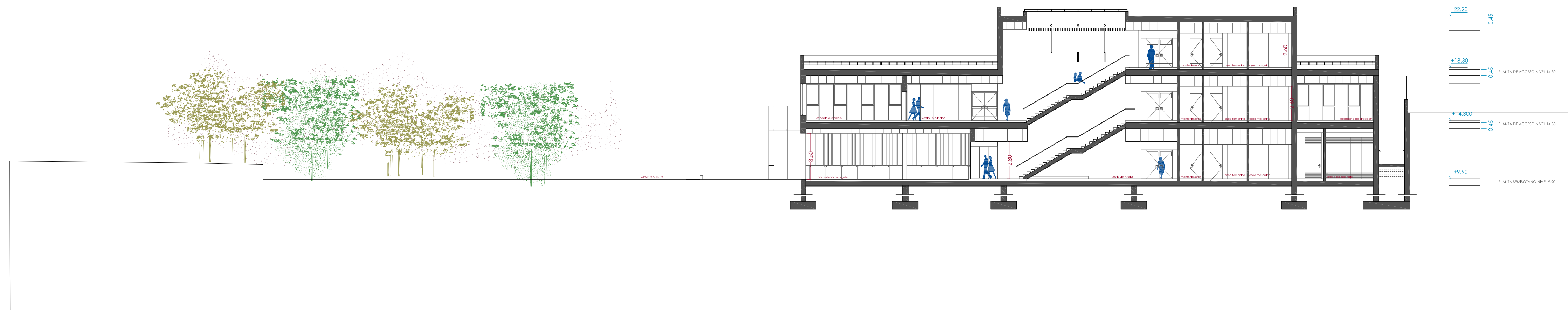
D-D'
