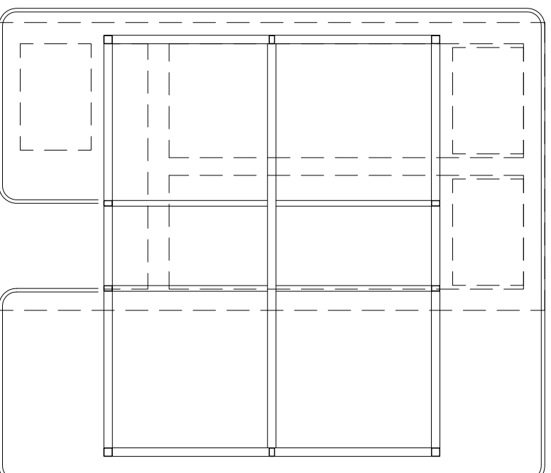
INVERNADERO: ESQUEMA ESTRUCTURAL DE CUBIERTA
