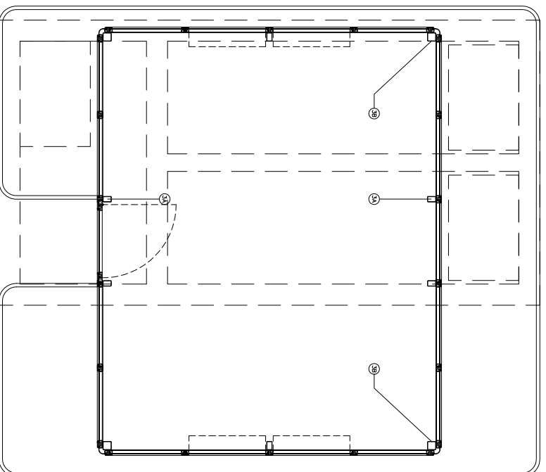
INVERNADERO: PLANTA
