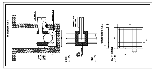
INSTALACIONES: DETALLES DE ACOMETIDAS e. 1/10-1/30
