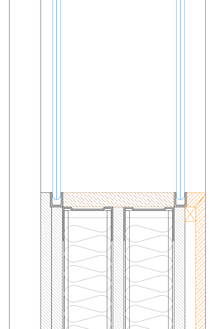
SECCIÓN VERTICAL ACRISTALAMIENTO F-1
