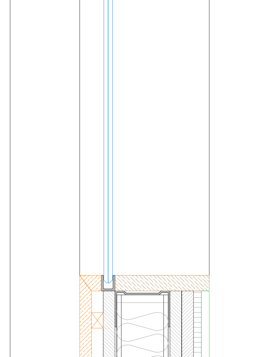
SECCIÓN VERTICAL VENTANA VI-10
