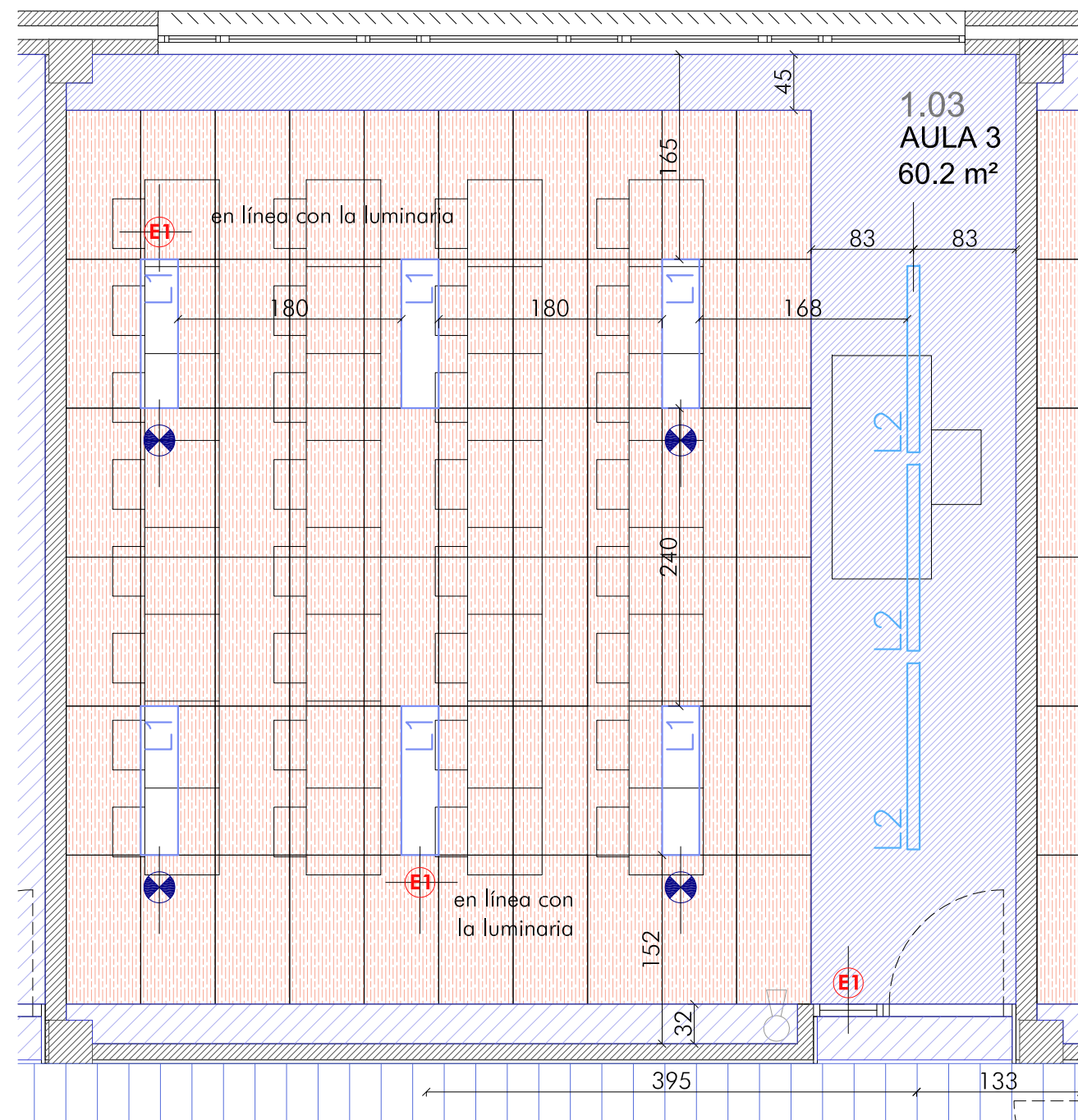
AULA TIPO - REPLANTEO TECHOS
