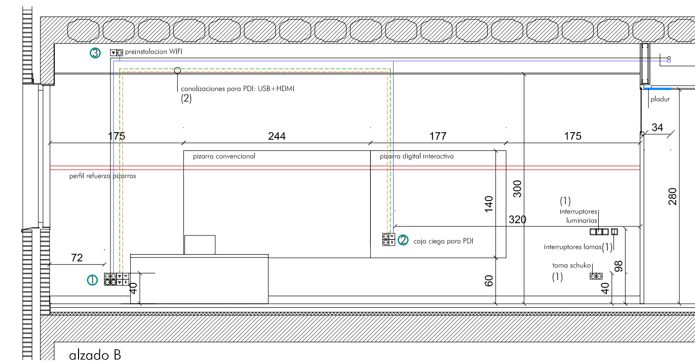
alzado B
