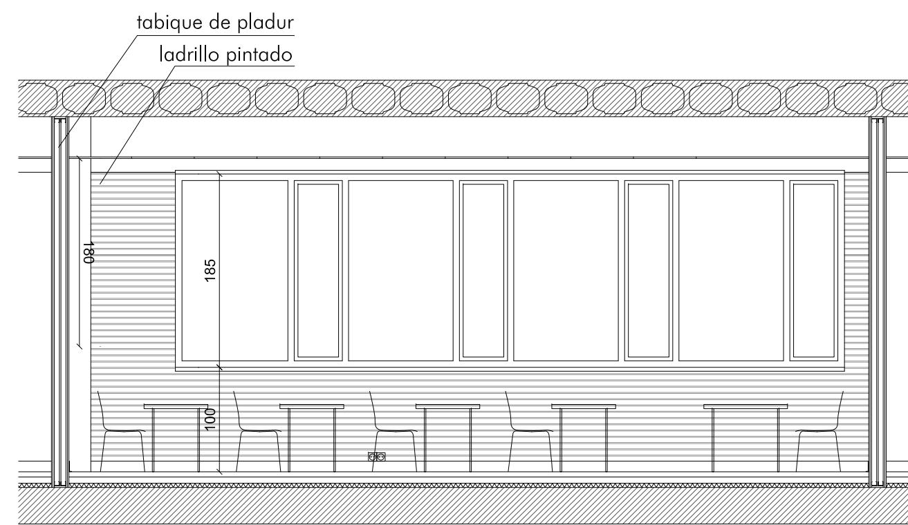
alzado A
