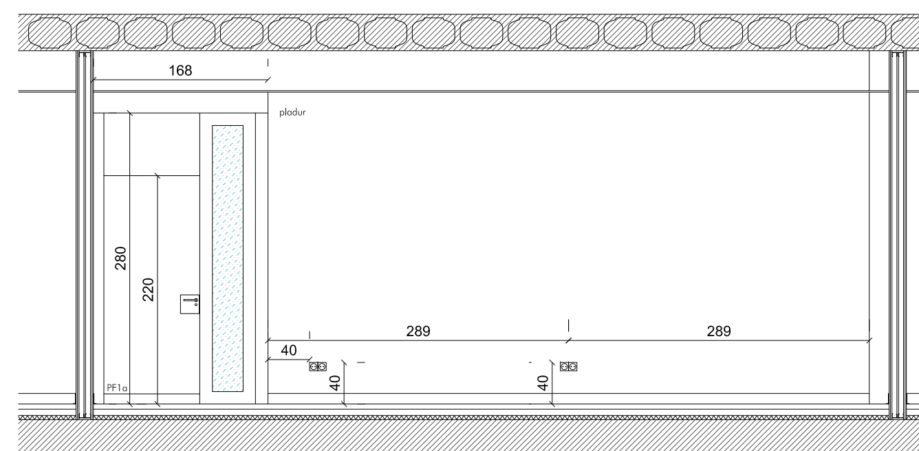
alzado C
