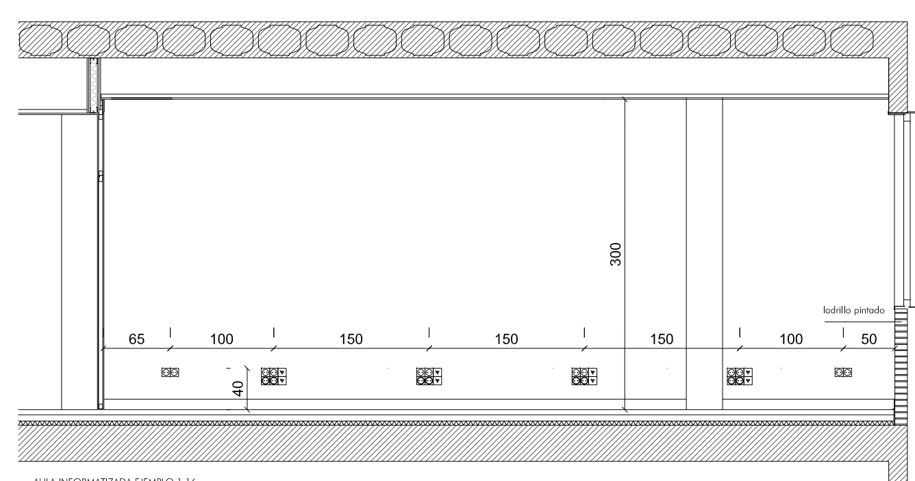
alzado C
