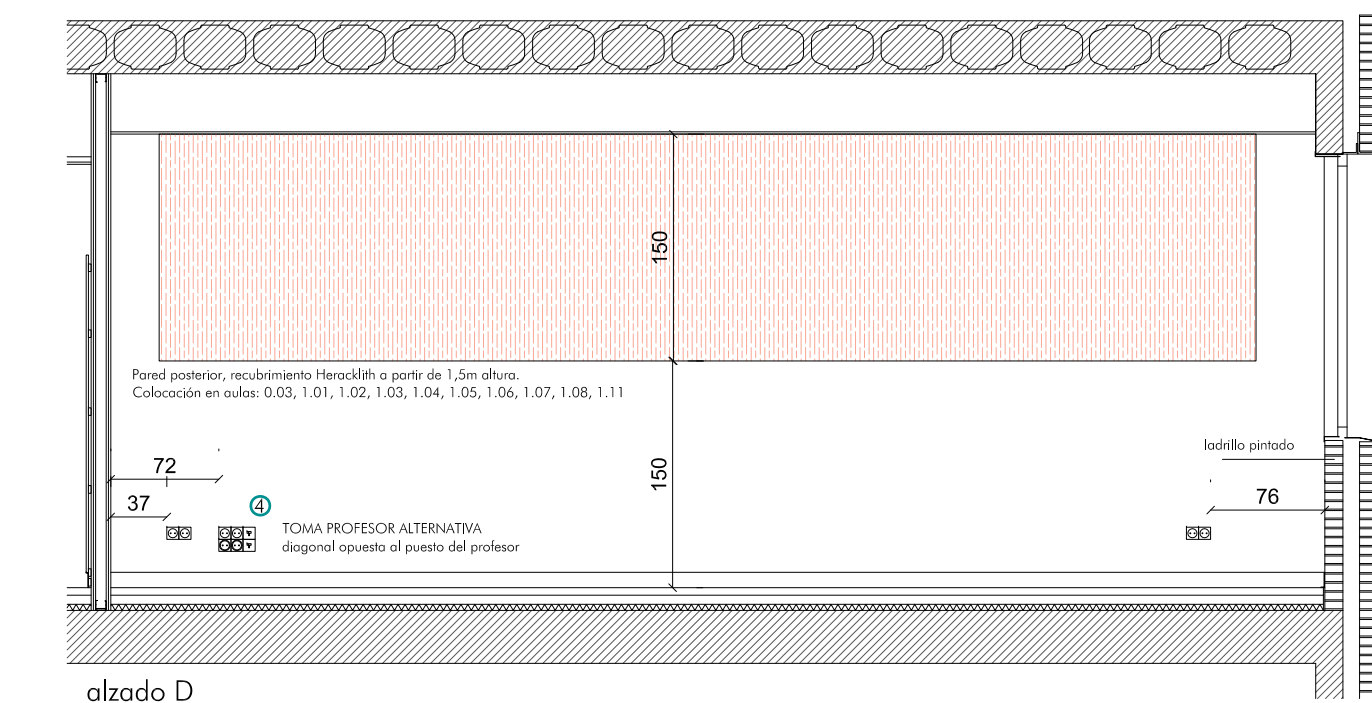
alzado D
