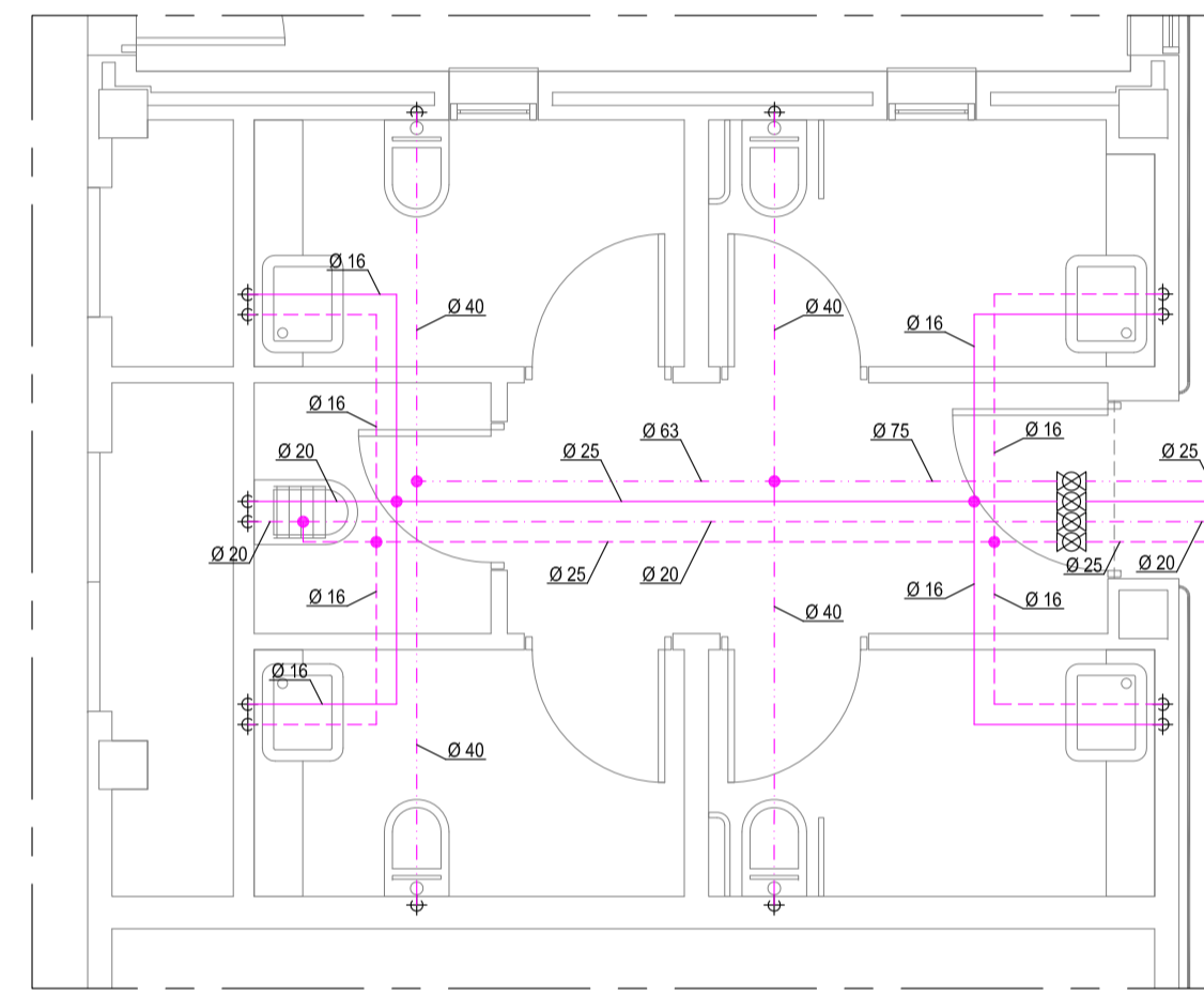
DETALLE TIPO 6
