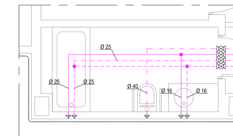
DETALLE TIPO 12
