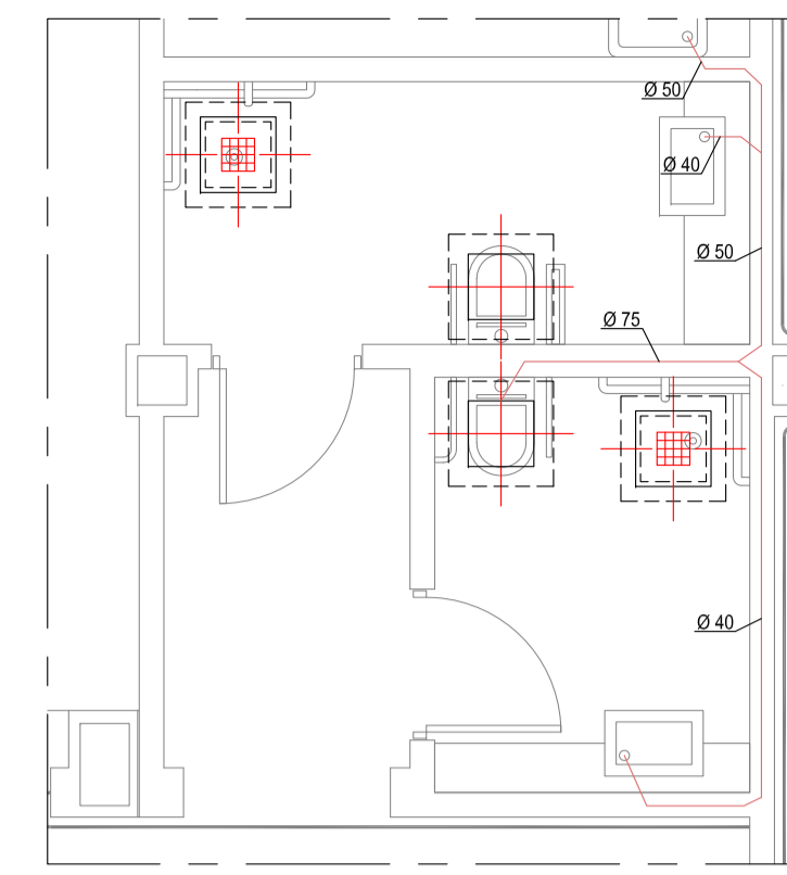
DETALLE TIPO 4
