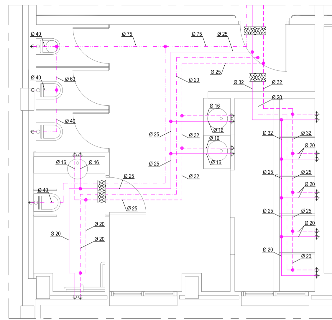
DETALLE TIPO 2
