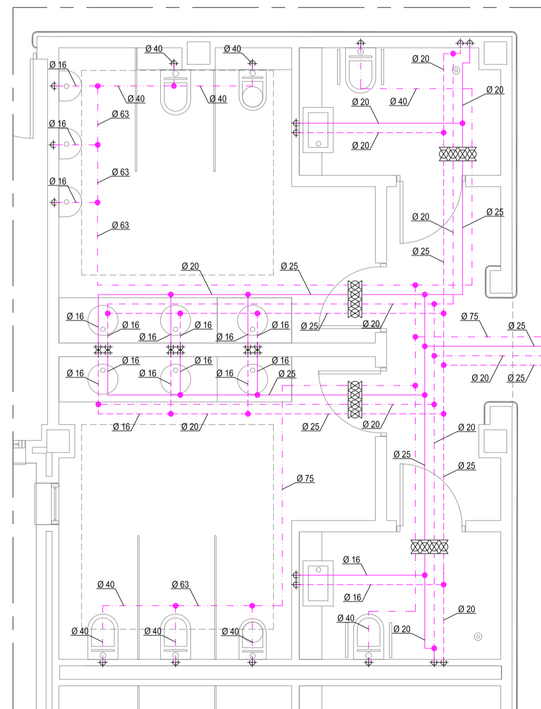
DETALLE TIPO 5
