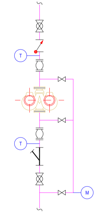
DETALLE CONEXION BOMBAS
