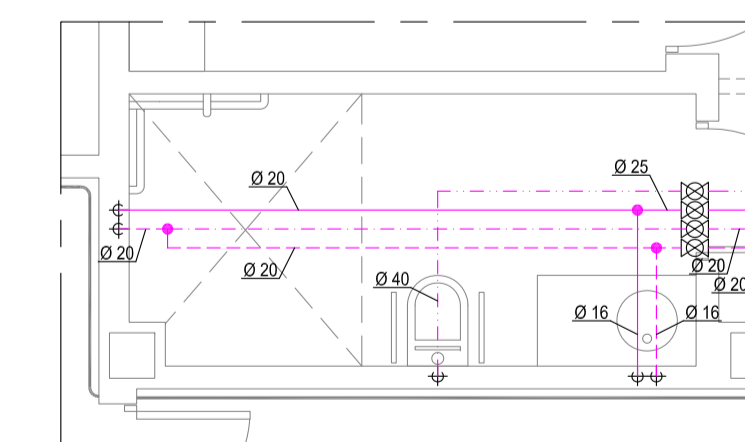
DETALLE TIPO 13
