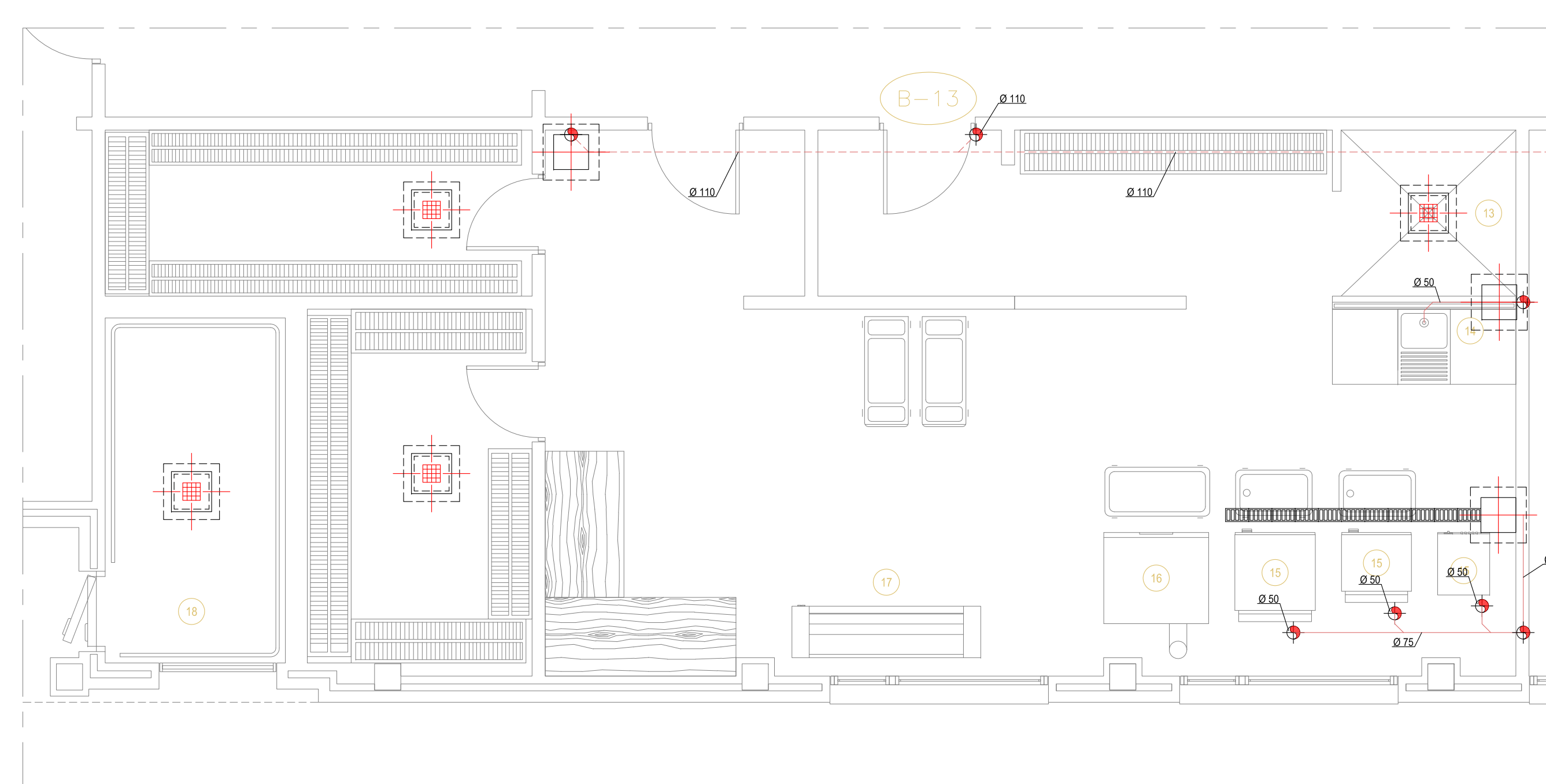
LAVANDERÍA (DESAGÜES)
