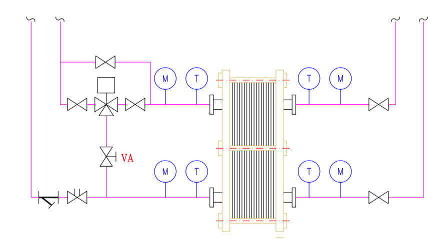
DETALLE CAMBIADORES
