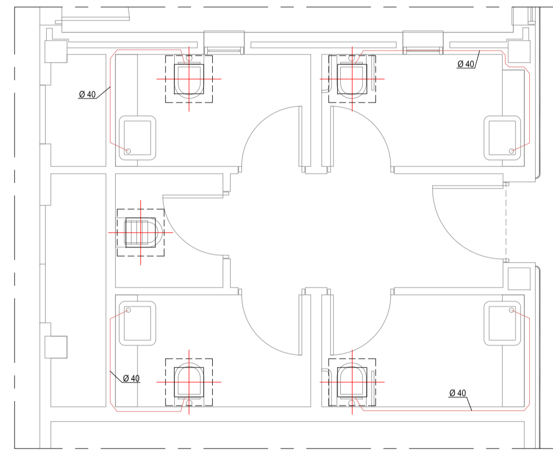
DETALLE TIPO 6
