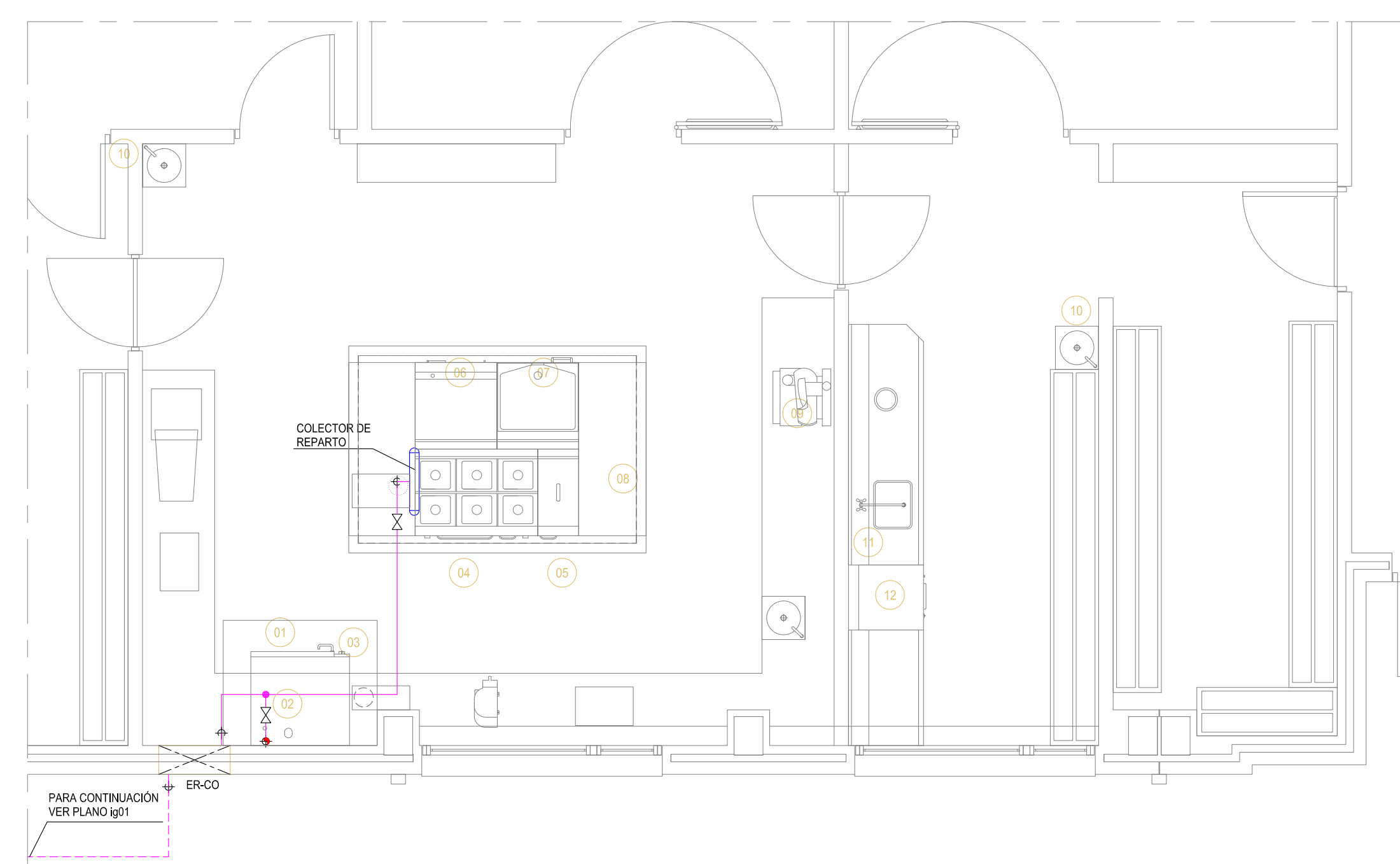
COCINA (GAS)
