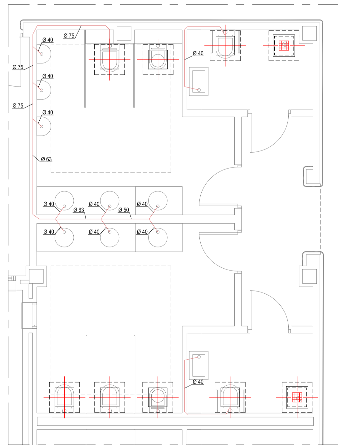
DETALLE TIPO 5
