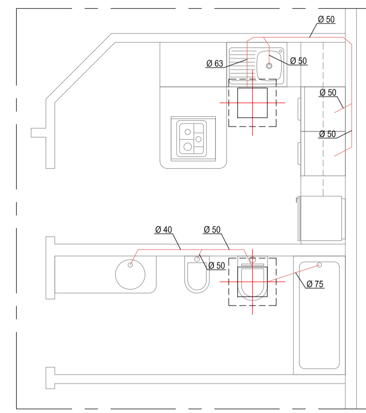
DETALLE TIPO 3
