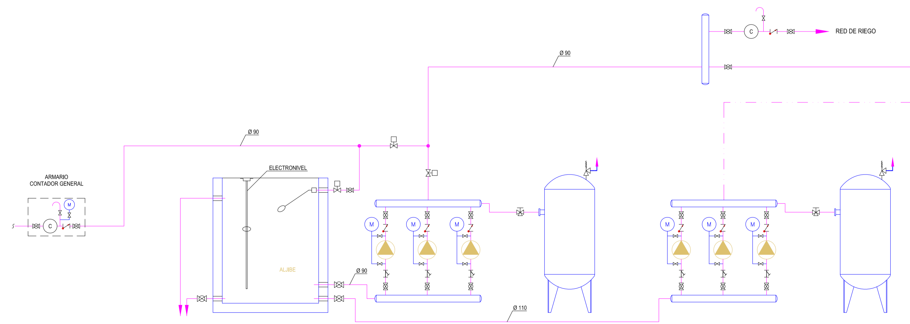
GRUPO DE PRESIÓN AGUA POTABLE
