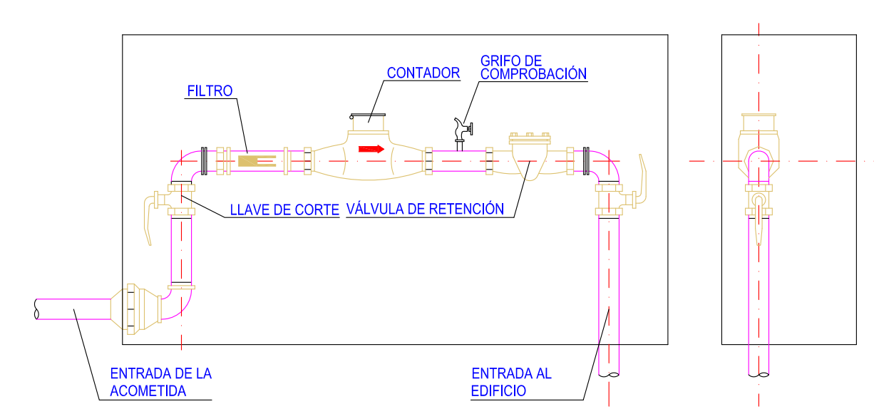
CONJUNTO DE ARMARIO CONTADOR GENERAL SIN ESCALA
