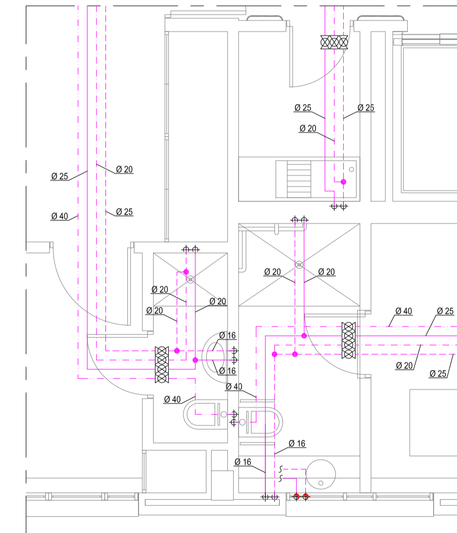
DETALLE TIPO 11
