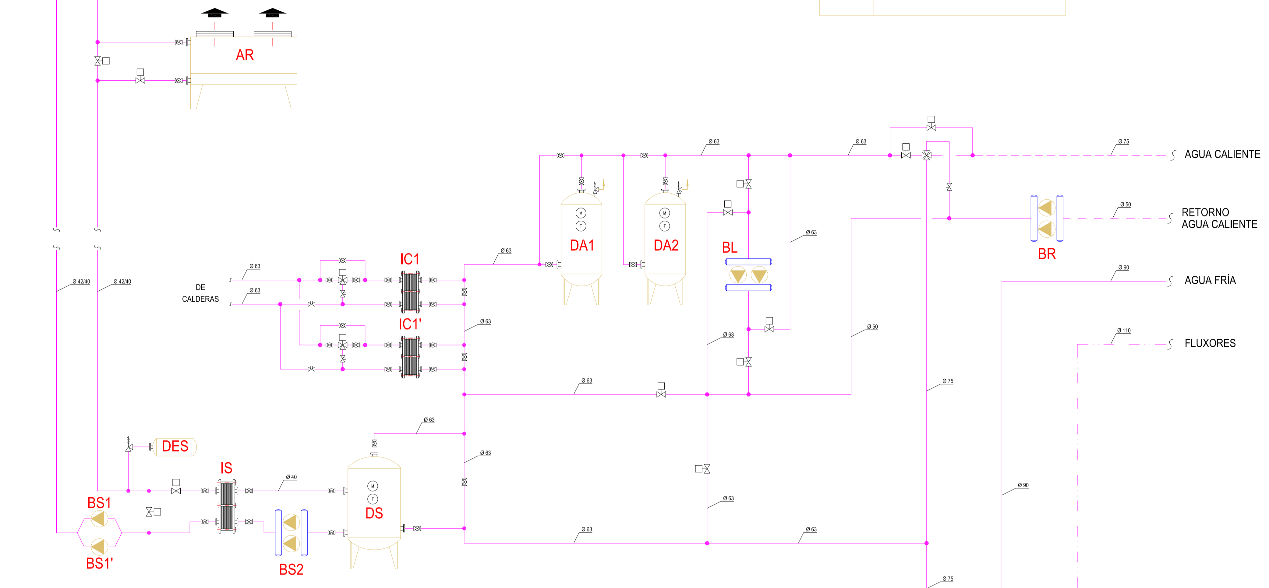
ESQUEMA DE PRODUCCIÓN A.C.S.
