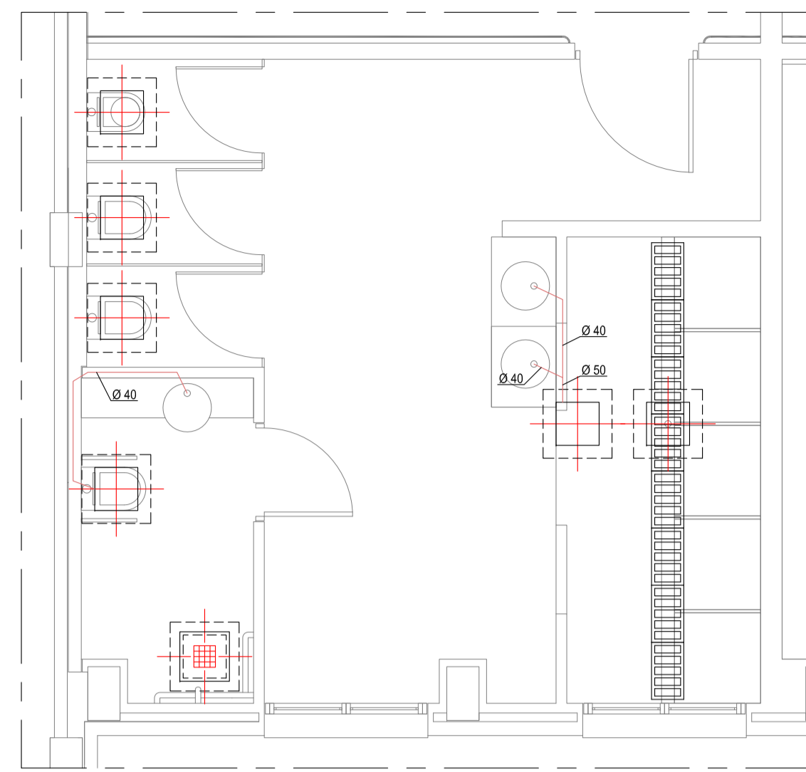
DETALLE TIPO 2
