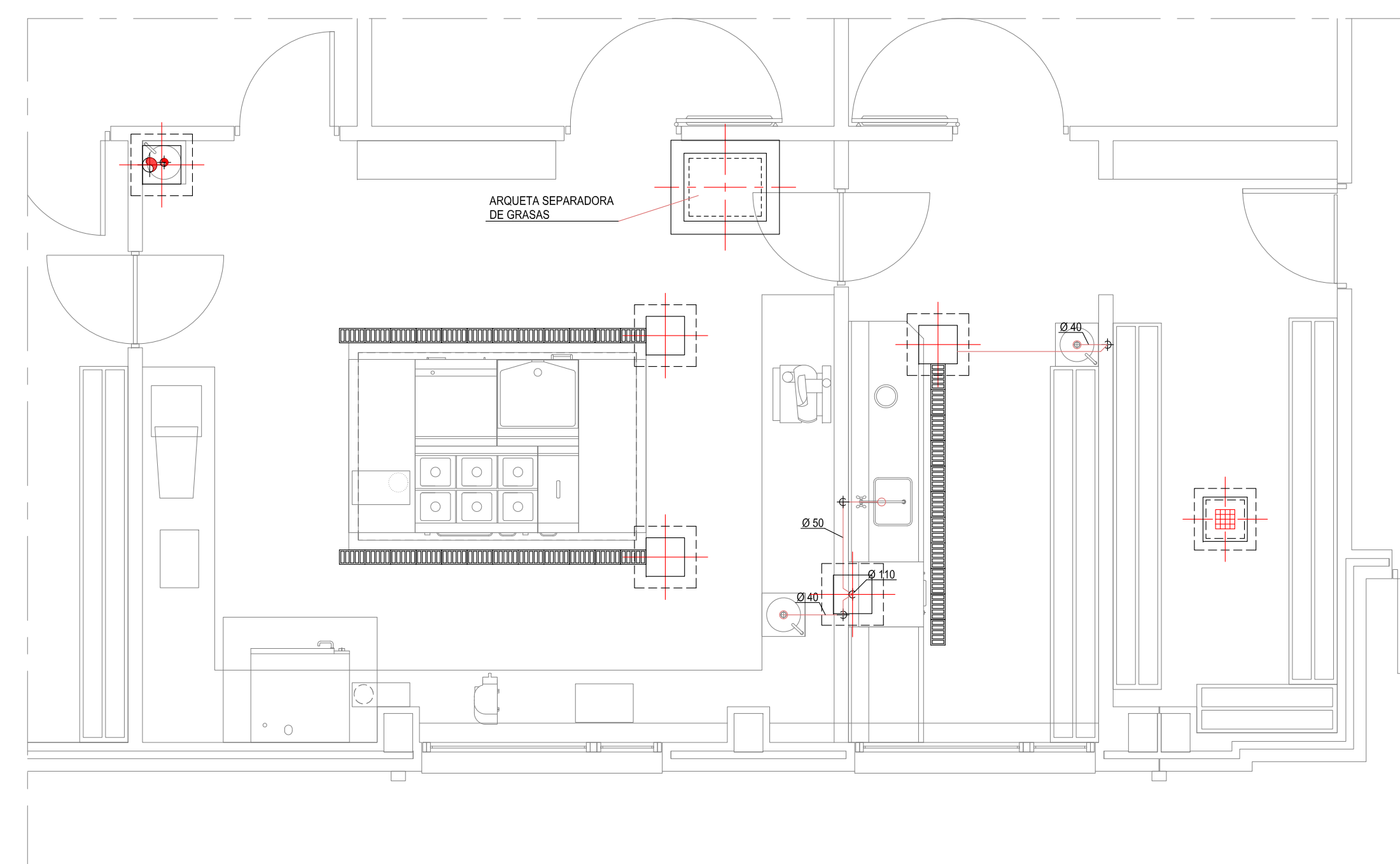
COCINA (DESAGÜES)
