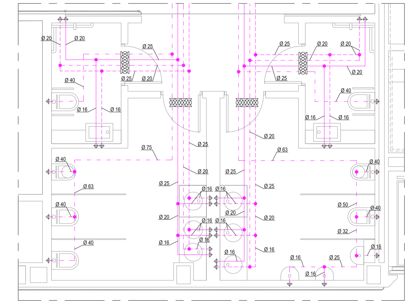
DETALLE TIPO 8
