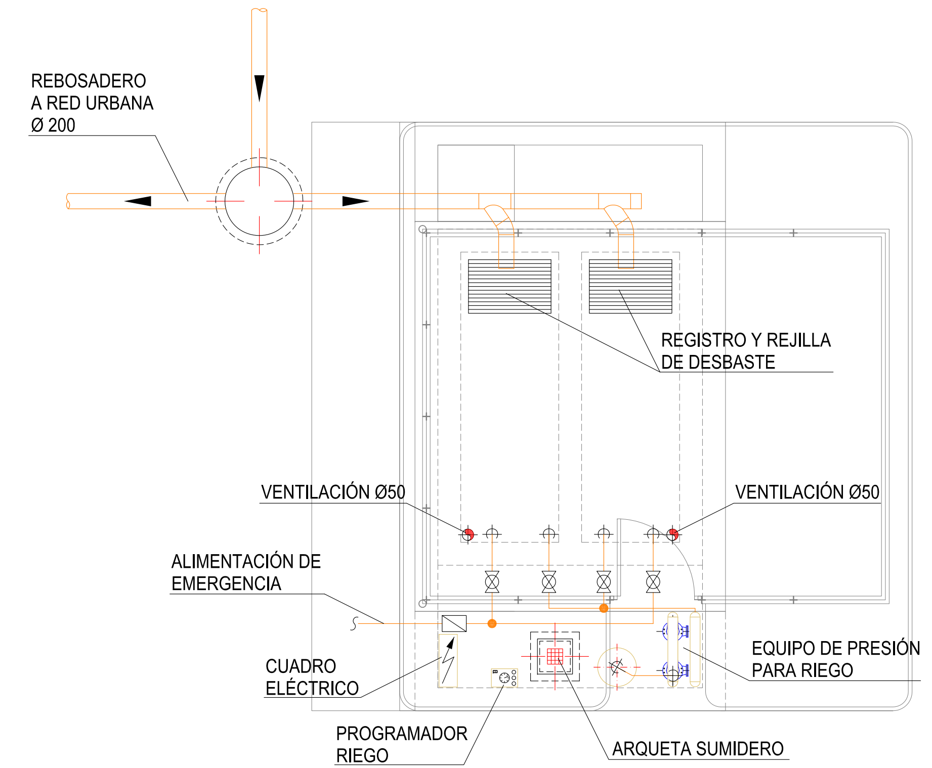
DETALLE ESTACIÓN DE BOMBEO PARA RIEGO RECOGIDA DE AGUAS PLUVIALES e: 1/50
