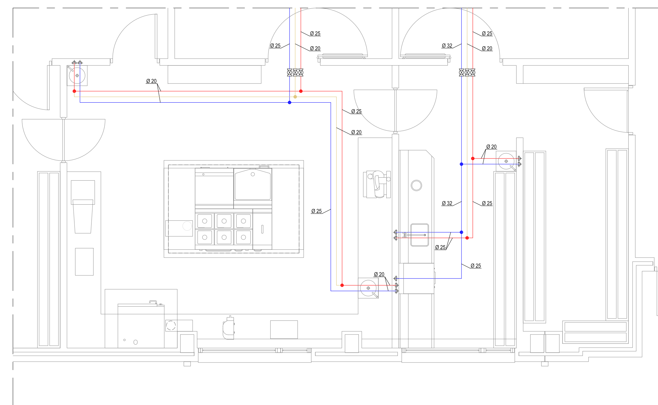
COCINA (AGUA)
